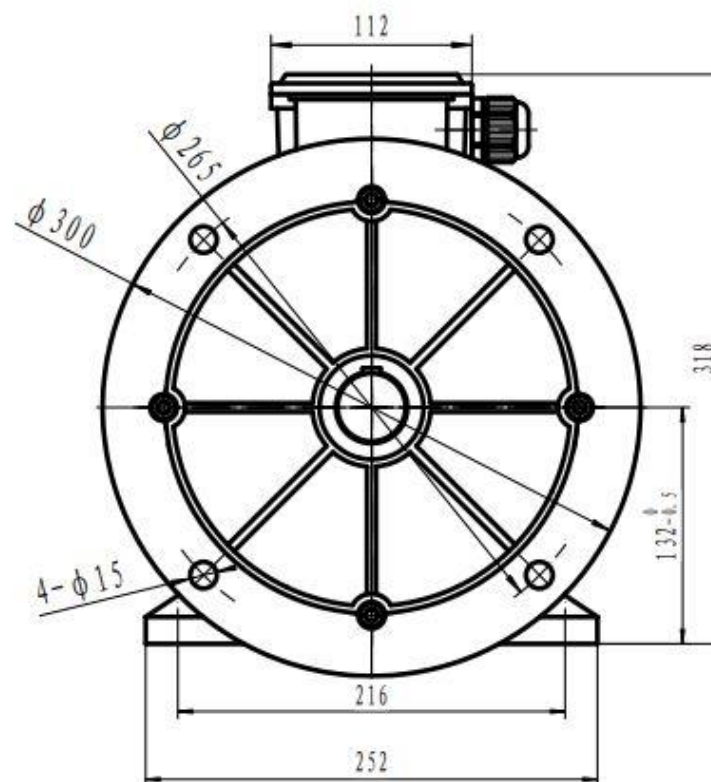
TECA BM 132 Frame B35
