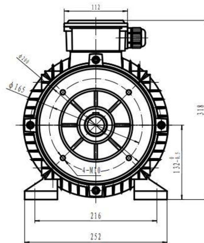
TECA BM 132 Frame B34
