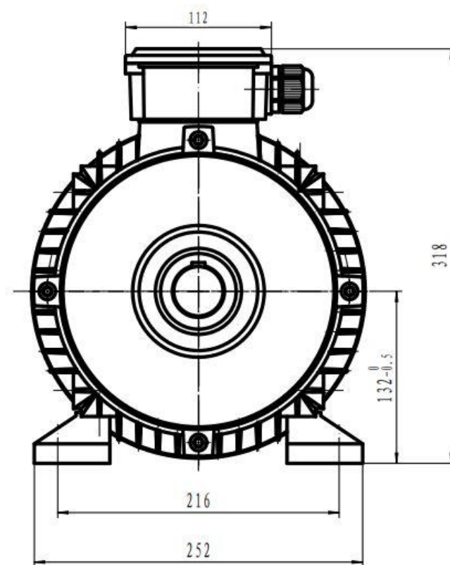
TECA BM 132 Frame B3
